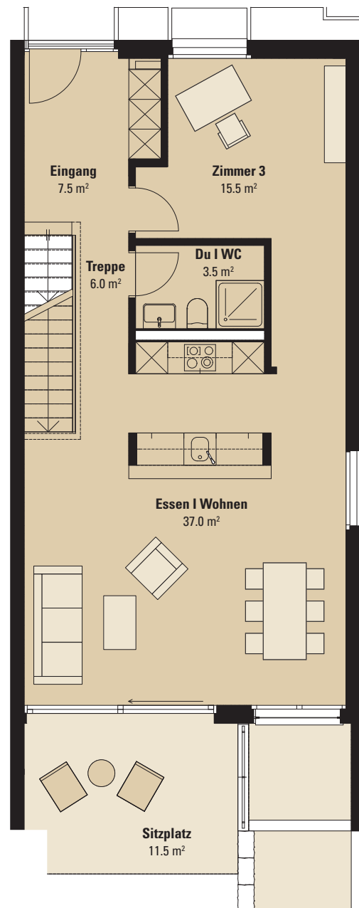
Erdgeschoss
