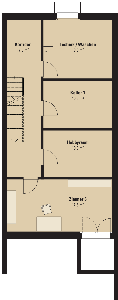
Untergeschoss
